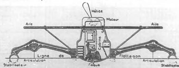
Croquis del aparato ideado por el ingeniero ucraniano.
